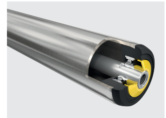
Rodillo transportador universal Serie 1700 heavy | página 76
