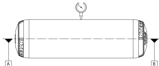
Fig.: Medición de la desviación de concentricidad
